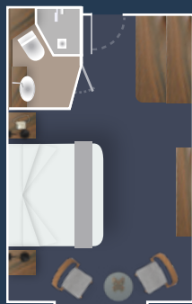
CABINA SUPERIOR 20,5 m2 220 sq. ft.
